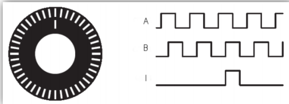
Figura 1: Ejemplo de disco ranurado y de señales en cuadratura junto con la señal de referencia, generadas por un encoder incremental.
