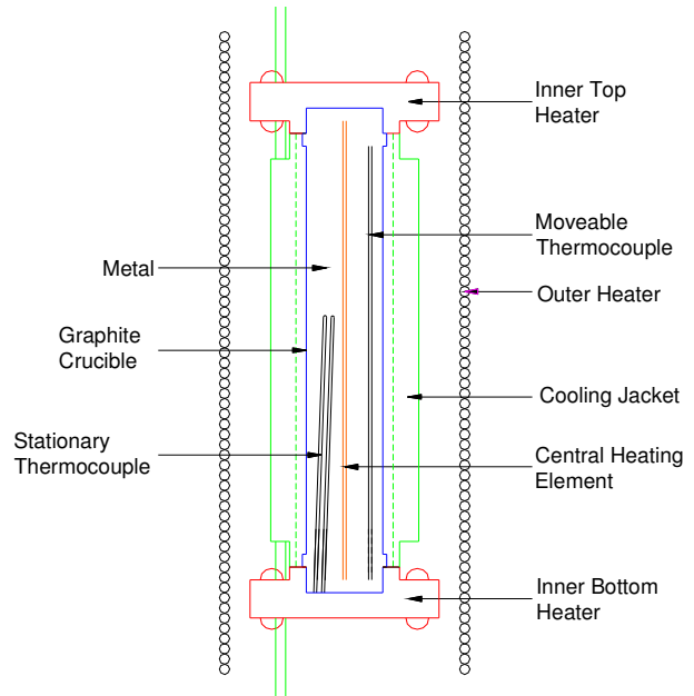
Fig. 6 El aparato de flujo de calor radial y sus componentes principales
