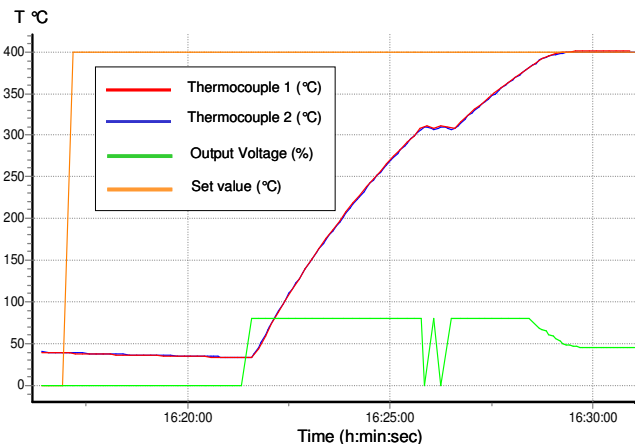
Fig. 9 Secuencia de optimización del control de temperatura a 400°C
