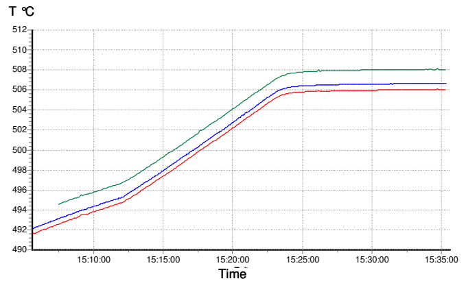
Fig. 8 Calibración de las termocuplas a la temperatura de líquidos. Tres termocuplas diferentes son calibradas y la diferencia en las temperaturas registradas son calculadas y corregidas.
