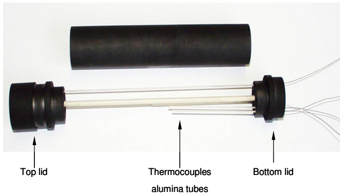
Fig. 7 La probeta se compone de un cilindro y dos tapas sellantes de grafito en los extremos superior e inferior con tubos cerámicos para aislar las termocuplas y el alambre resistivo axial.
