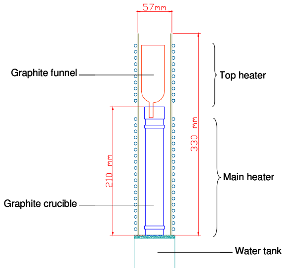
Fig. 5 El sistema de solidificación direccional conteniendo la probeta de grafito.
