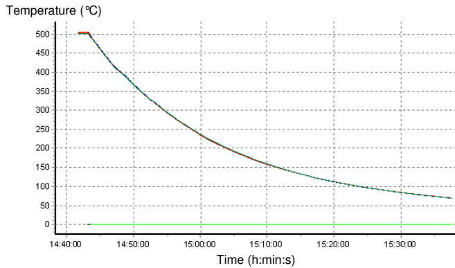
Fig. 10 Velocidad de enfriamiento registrada por el controlador térmico.
