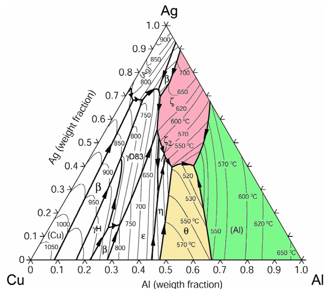
Fig. 1 Diagrama de equilibrio para el sistema Al-Cu-Ag resaltando las fases alfa, Teta y Zeta ( \alpha , \theta , y \zeta ) [2].
