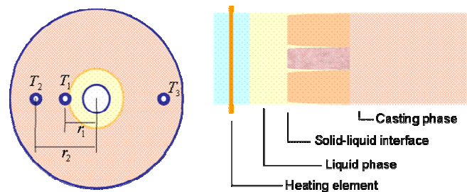
Fig. 11 Definición de los términos usados en el cálculo de K_S y G_S
