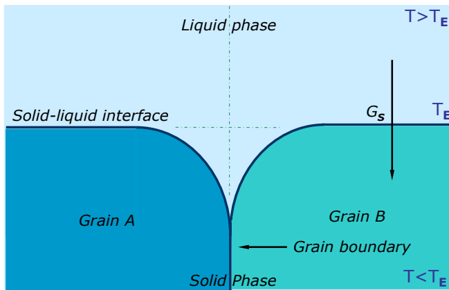
Fig. 2. Ilustración de una frontera de grano formada en la interfase sólida-líquida en equilibrio y la descripción del gradiente de temperatura y las temperaturas en la fase líquida, sólida y en la interfase plana.
