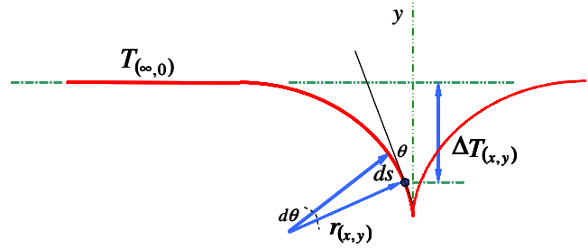
Fig. 3. Se ilustra el perfil de una frontera de grano describiendo las coordenadas y y \theta y la relación entre la curvatura en un punto cualquiera y el enfriamiento entre la línea de interfase plana y el punto descrito.
