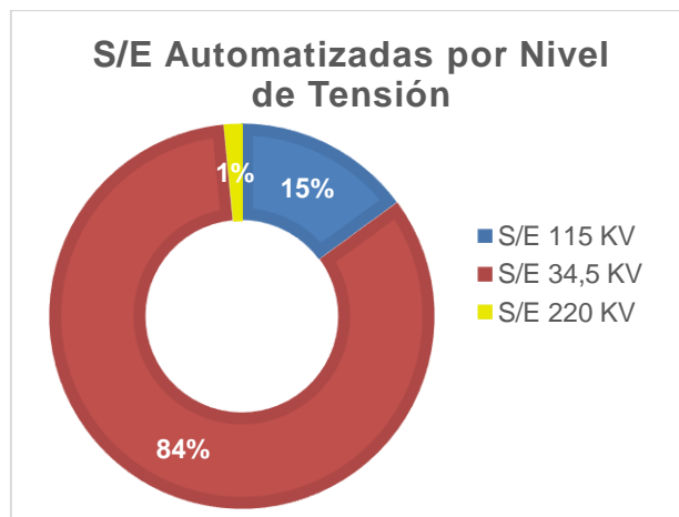
Figura 20. Distribución de subestaciones automatizadas por nivel de tensión.
